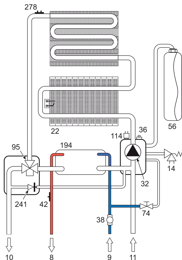
fig. 20 - Circuito sanitario
