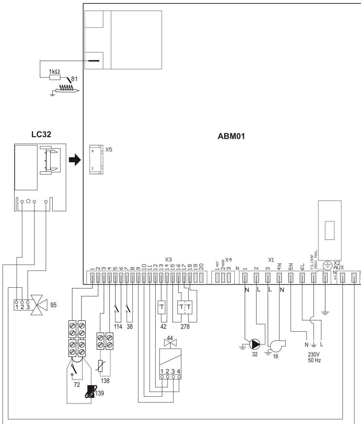
fig. 23 - Circuito eléctrico
