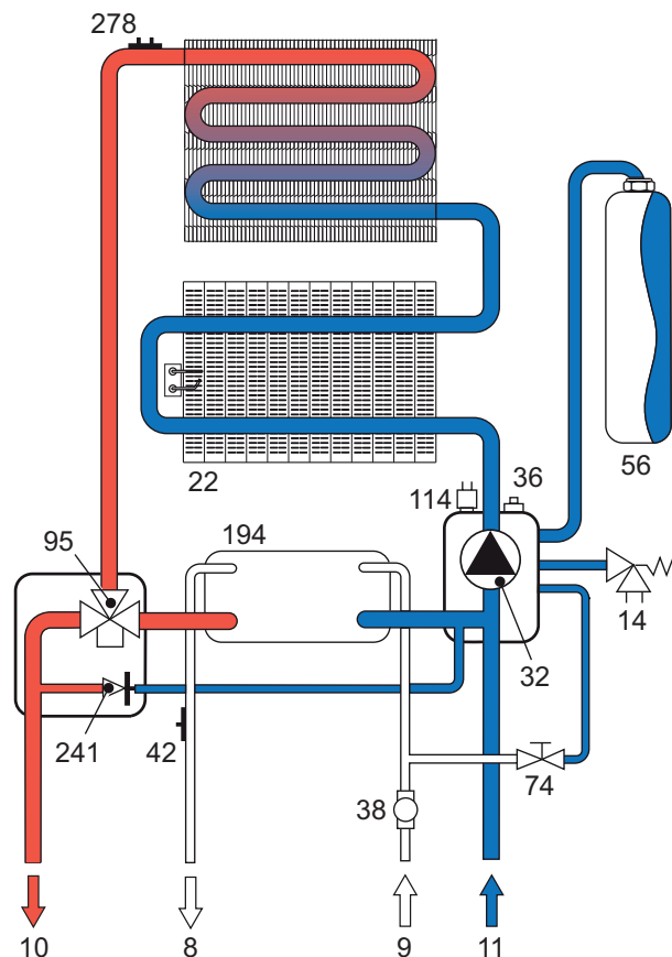
fig. 19 - Circuito calefacción
