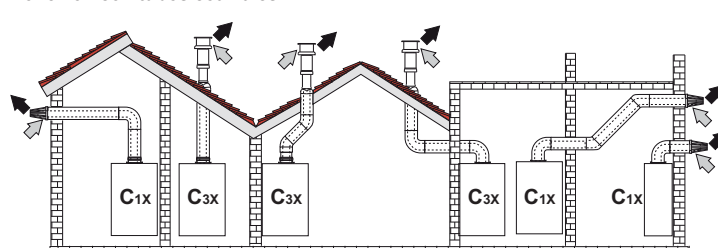
fig. 9 - Ejemplos de conexión con tubos coaxiales (⇐ = aire / ⇨ = humos)
